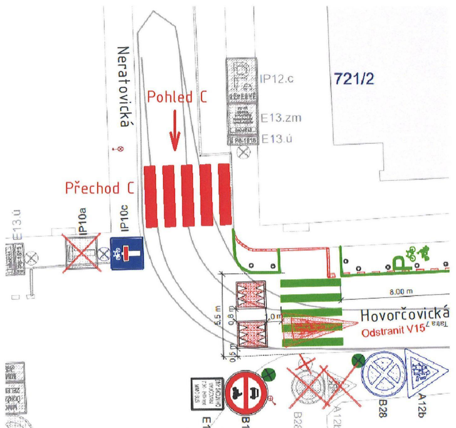
Obr. P.2-1 Návrh přechodu C
